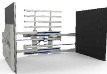
DOZENKLEM Capaciteit tot 2200 kg
